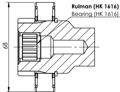
KESİT A-A ÖLÇEK 1 : 1.5
