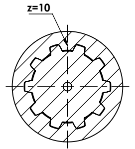
KESİT B-B ÖLÇEK 1 : 1.5
